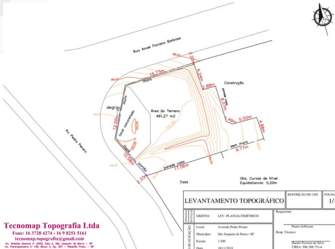
Figura 7 – Levantamento Planialtimétrico
